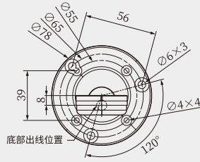
底座安装孔位
